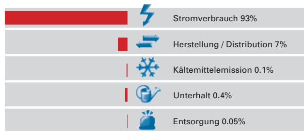
Umweltbelastung Tumbler während Geräte-Lebensdauer
